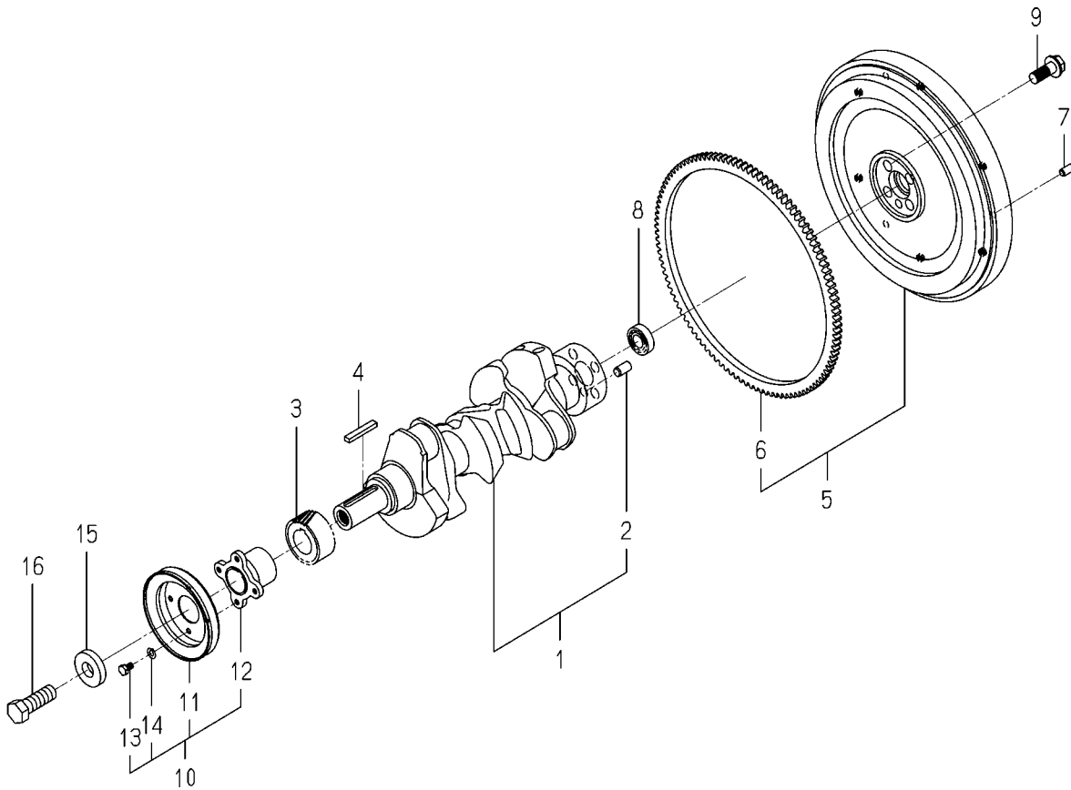
FIG. 15 CRANK SHAFT
