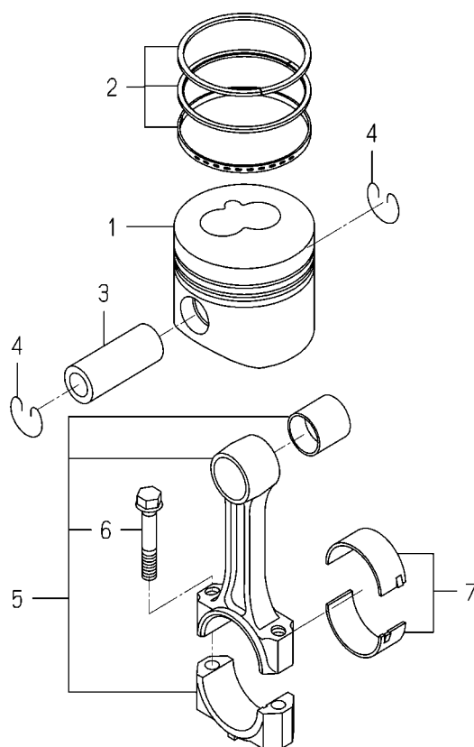
FIG. 13 PISTON
